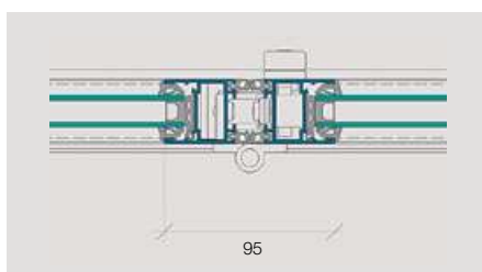
Sezione centrale con chiusura, apertura verso l'interno
