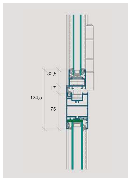
Parapetto (vetratura fissa) con parete a libro
