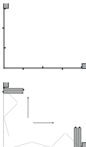
Sistema angolare senza montanti a 90°
