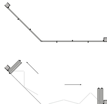
Sistema angolare senza montanti a 135°
