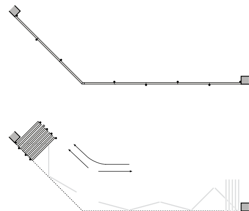
Sistema a raggio senza montanti a 135°
