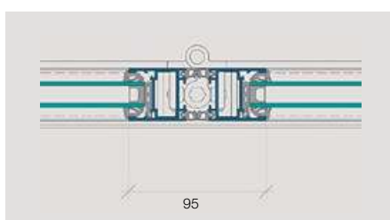
Sezione centrale con nastro interno
