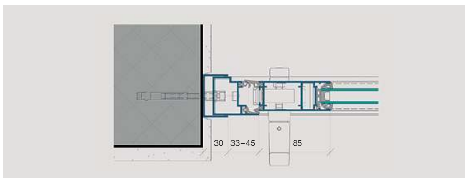
Sezione orizzontale con anta manovrabile, apertura verso l'interno
